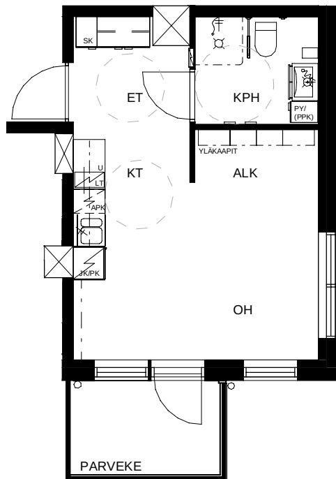
Kerros 4
