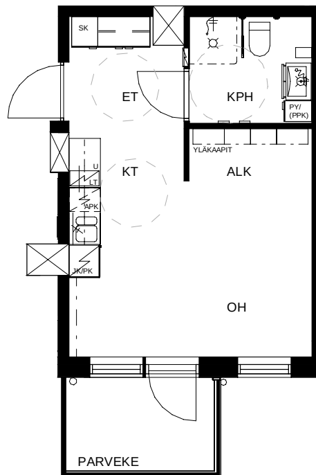
Kerros 4
